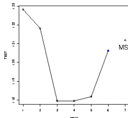
Test MSE
